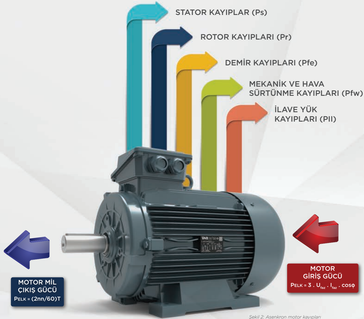
Şekil 2: Asenkron motor kayıpları
