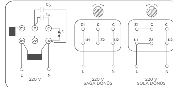
Şekil 16: 1 Fazlı kalkış ve daimi kondansatörlü motorların klemens bağlantısı
